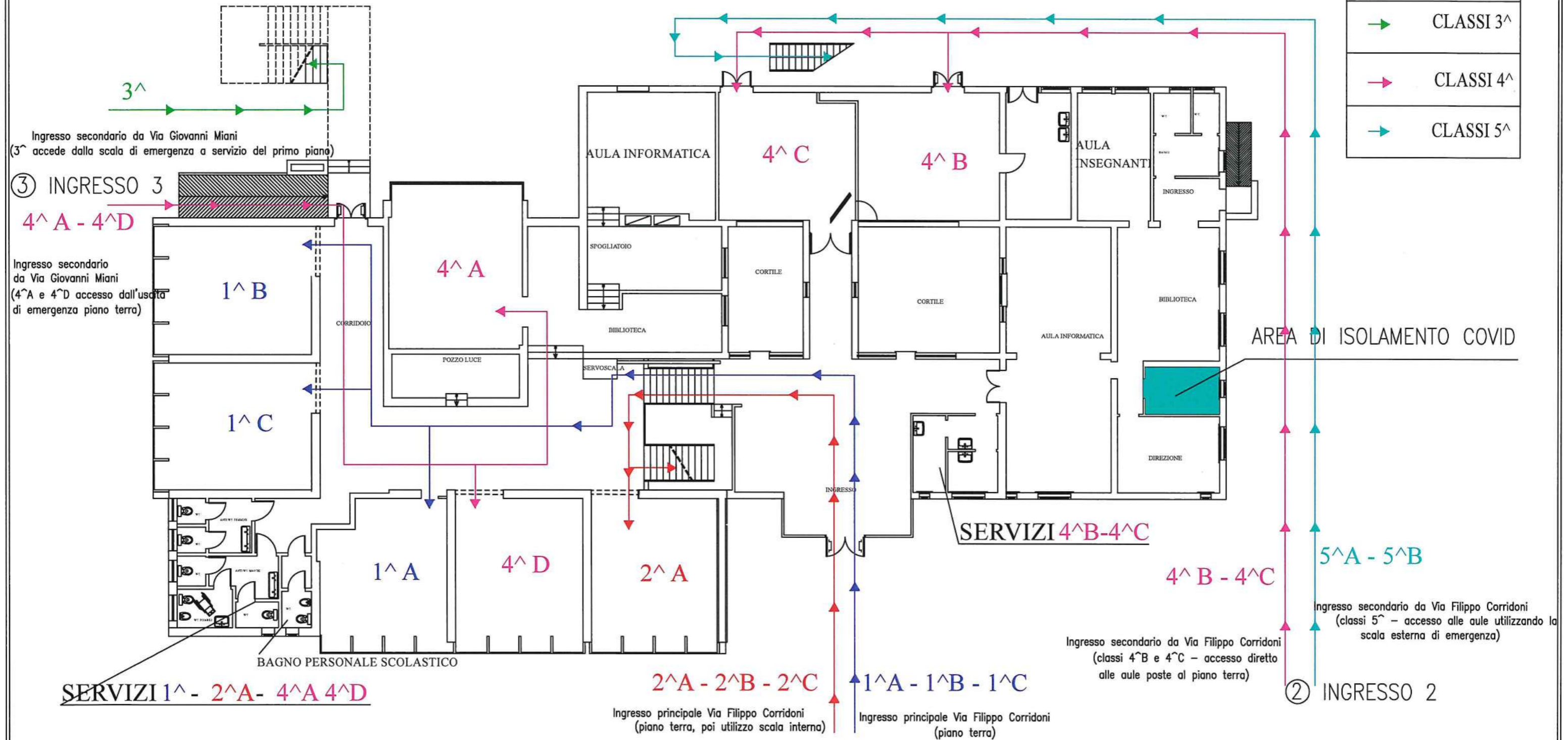
PIANTA PIANO TERRA E RIALZATO
